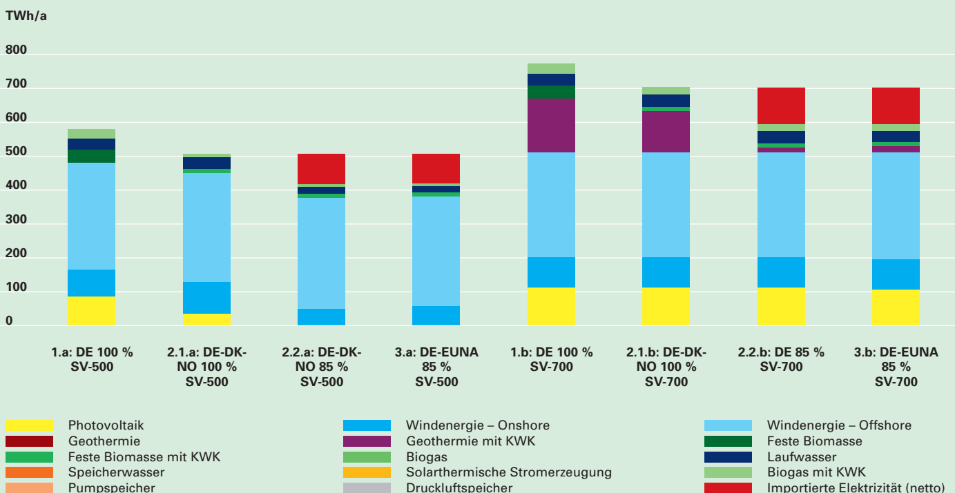
Abbildung 1: Elektrizitätserzeugung in Deutschland und Nettoimporte im Jahr 2050 (Quelle: SRU/SG 2011-1/Abb. 0-1)
